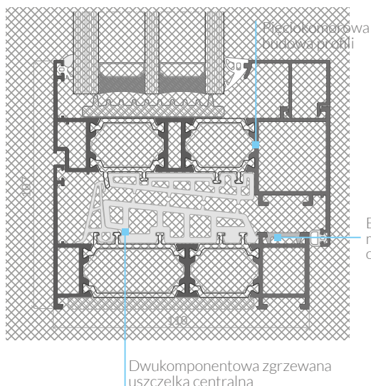
Przekrój przez okno otwierane
