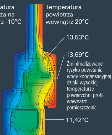
Corona AS 60 Przebieg izoterm
